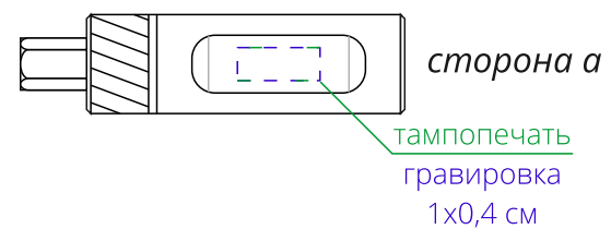
магнитный держатель 1
