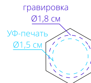
шестигранная панель
