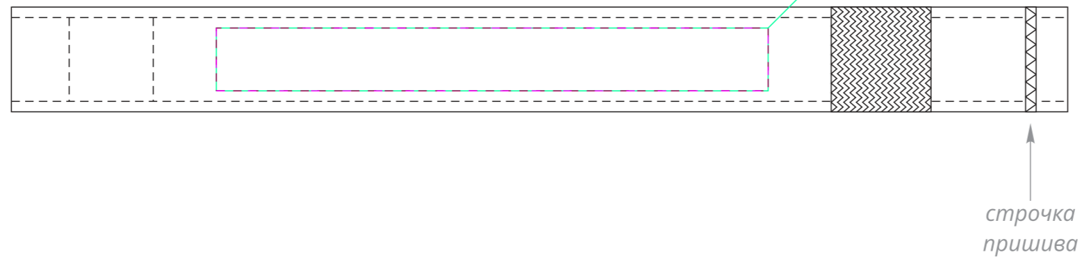
хлястик (зонт в закрытом виде, ручка зонта направлена вниз) M1:1
