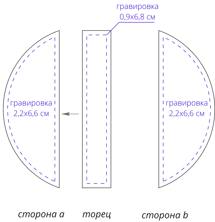
полукруглая деталь (36 шт.)
